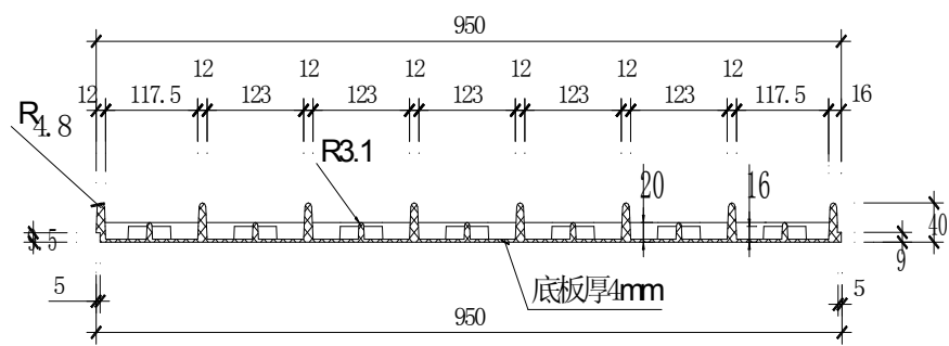
1-1剖面
