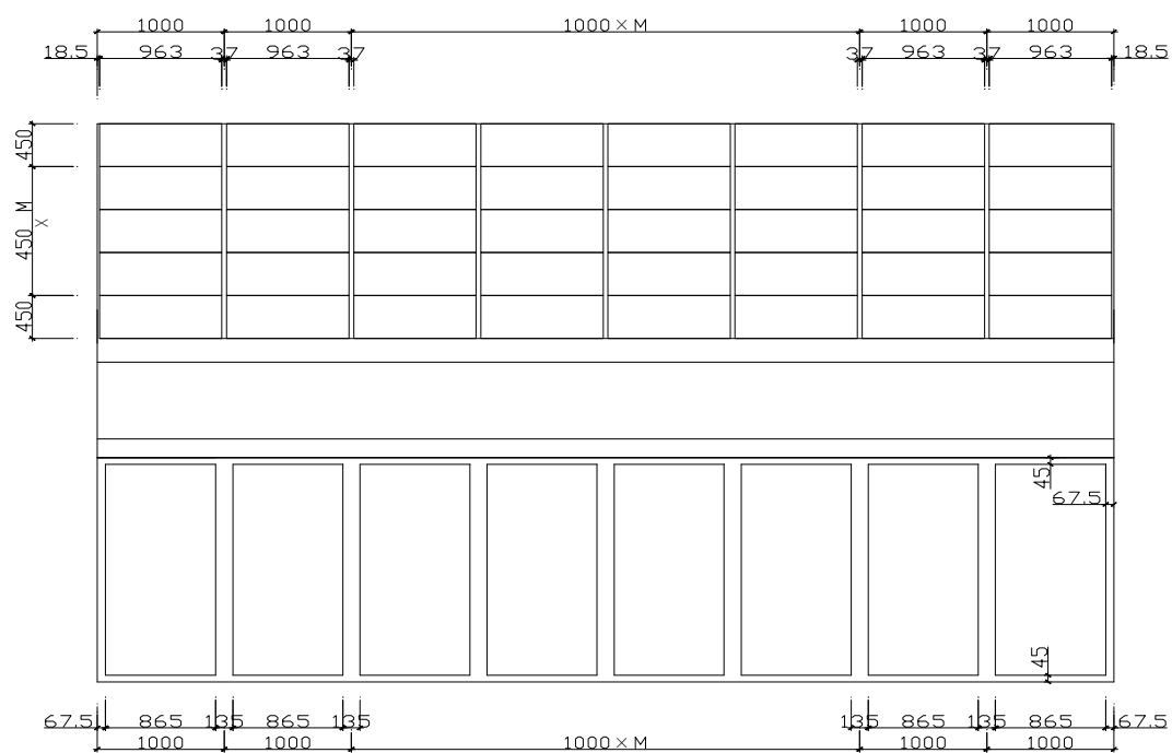
B 型模板平面图
