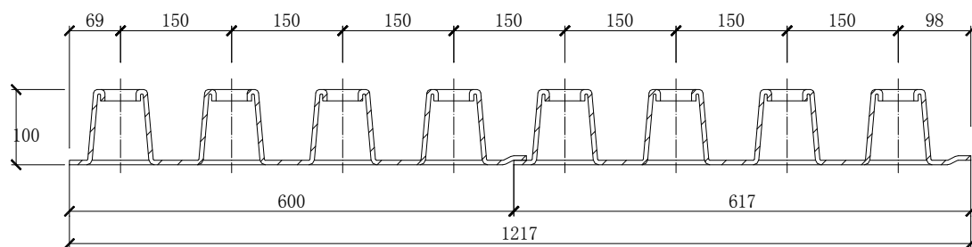
1 - 1 剖面（二块叠合）
