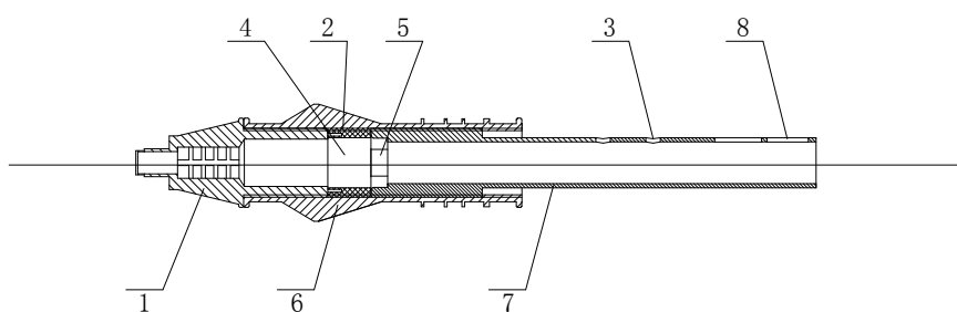
图4.4.1-2 可调式滤头 QSK-W-2型
