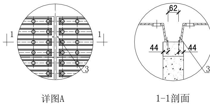
图 4.3.9 滤板支撑、边梁平面剖面图
