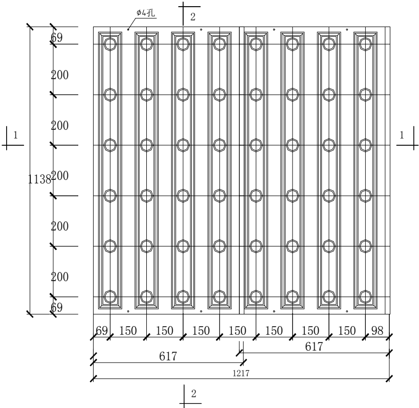
平面（二块叠合）
