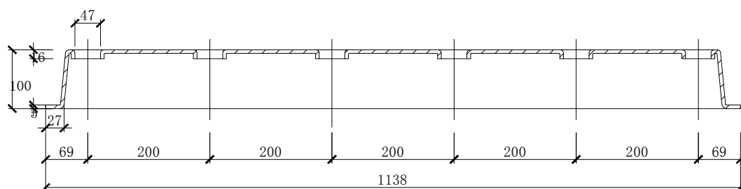
2-2剖面
