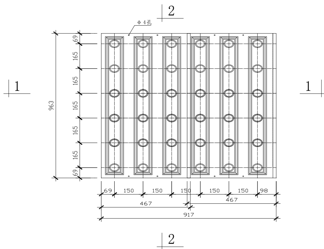
平面图 （两块叠和）
