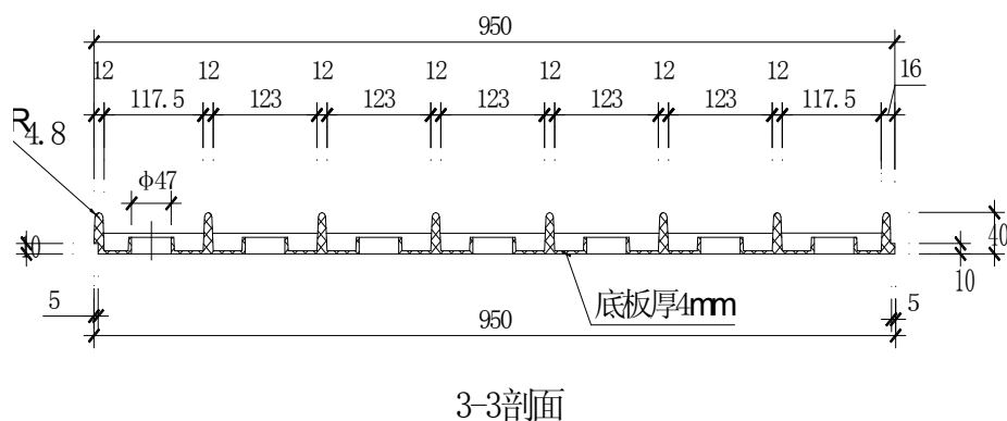
图 4.1.4 C 型模板平面、剖面图
