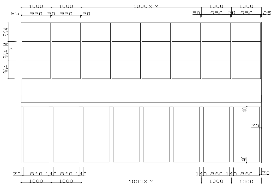
C 型模板平面图
