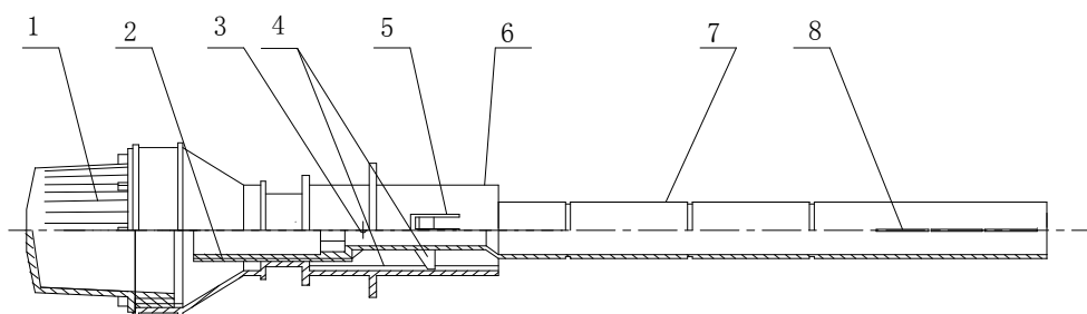
图 4.4.1-1 可调式滤头 QSK-W-1 型
